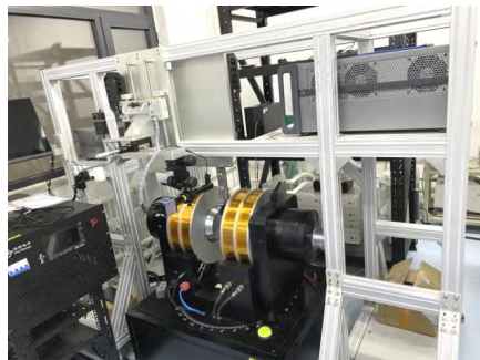
DMH磁场探针台
