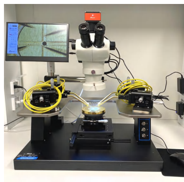
DM系列基础型探针台
