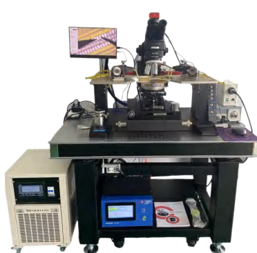
DH系列综合型探针台
