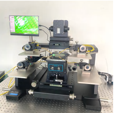
DSH双面型探针台
