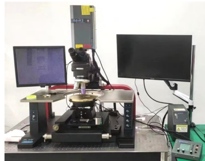
FA失效分析探针台
