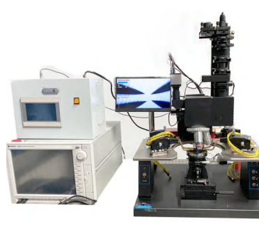
DG光电流探针台
