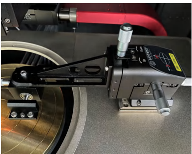
微分头型射频探针座
