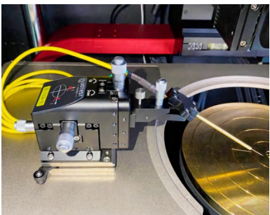
微分头型探针座
