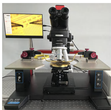
DN系列增强型探针台
