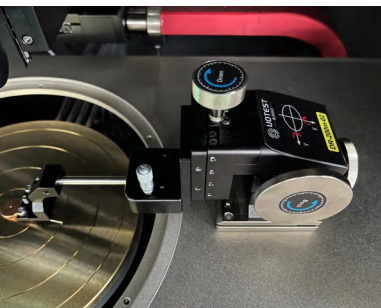
丝杆型射频探针座
